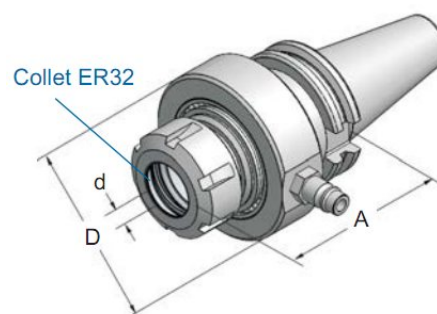
DIN 69871
